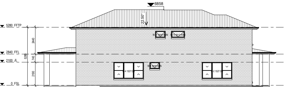
Elevation 2 1 : 100
