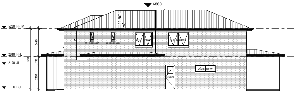
Elevation 1 1 : 100
