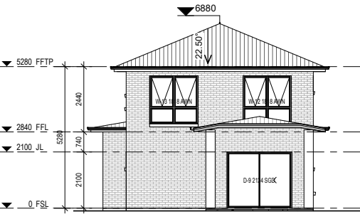
Elevation 4 1 : 100
