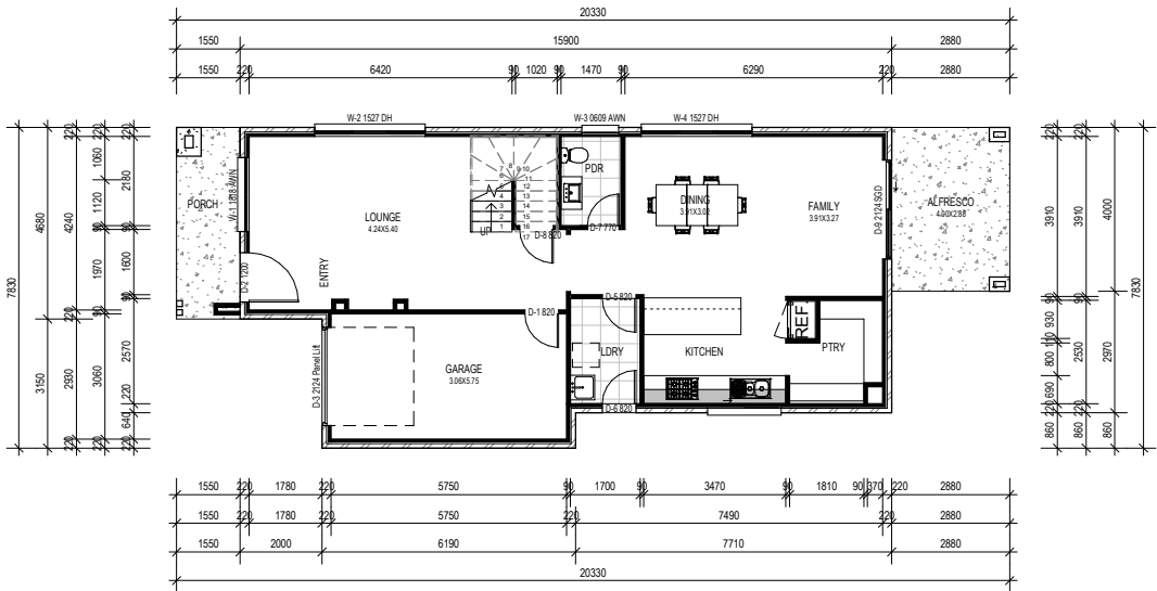
Floor Plan 1 : 100
